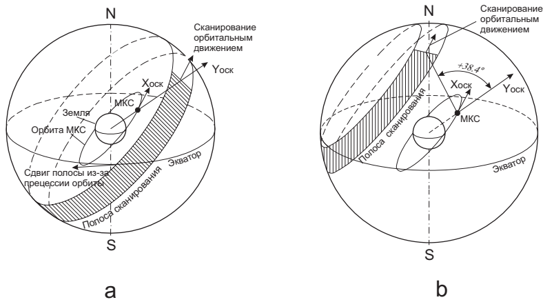
Рис. 1. (а) Сканирование неба в основной ориентации инструмента — ось телескопа лежит в плоскости орбиты. (б) Ось телескопа смещена на 38.4^\circ к северу, полоса сканирования проходит через северный полюс мира
